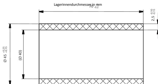
Abbildung 1: Beispiel für die Tolerierung einer Lagerbuchse
